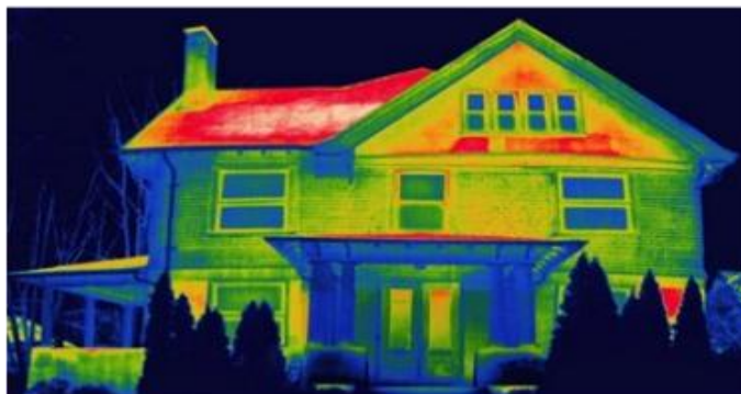
Obr. 29 Termovizní měření tepelných ztrát (zdroj: Elogy s.r.o.)
